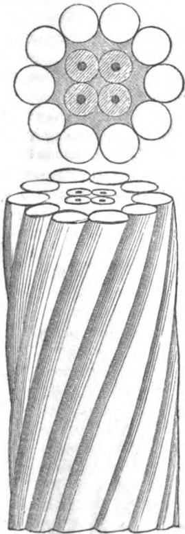
Fig. 2.—Dover Cable.
