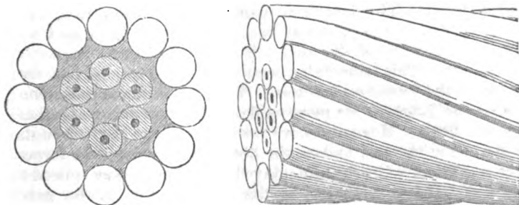
Fig. 14.—Mediterranean Cable.
