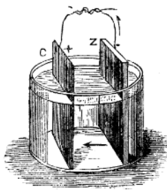
FIG. 1.—THE VOLTAIC PAIR.
