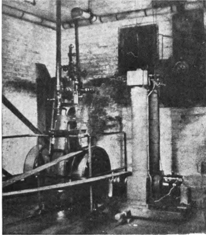
DYNAMOS, HINDS, KETCHUM & CO. 1881
