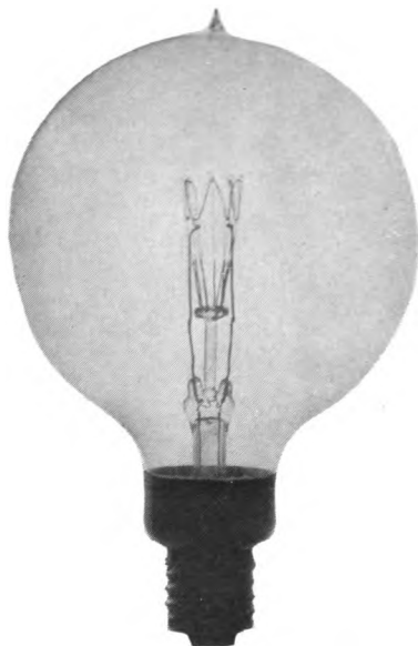
GAS-FILLED TUNGSTEN FILAMENT LAMP, 1913
