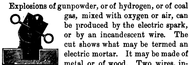
FIG. 43. ELECTRIC MORTAR.
