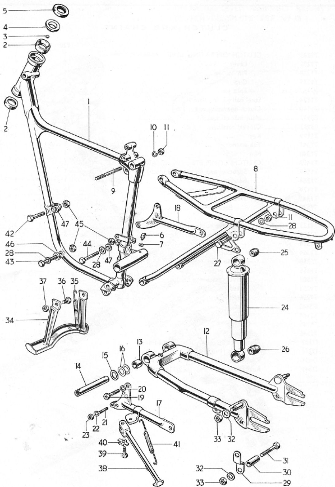
Fig. 8. FRAME COMPLETE
