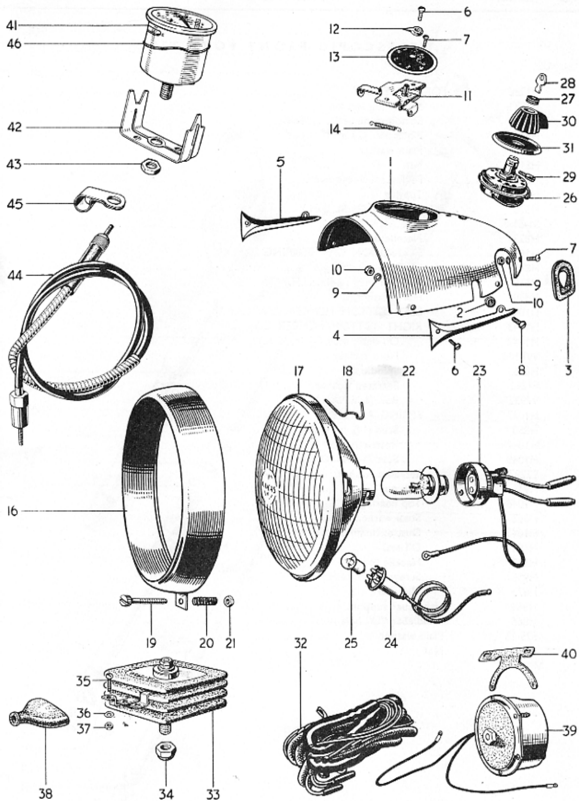
Fig. 11. NACELLE, HEADLAMP, Etc.
